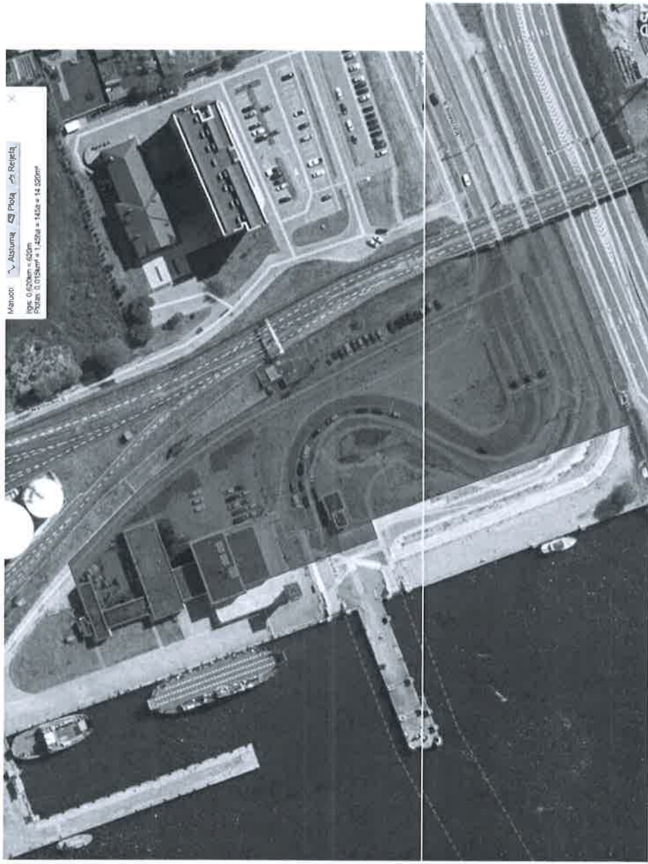
1 pav. AB "Smiltynės perkėla" 1,45 ha teritorija , nuo kurios paviršinės nuotekos surenkamos, apvalomos ir išleidžiamos į Kuršių marias
